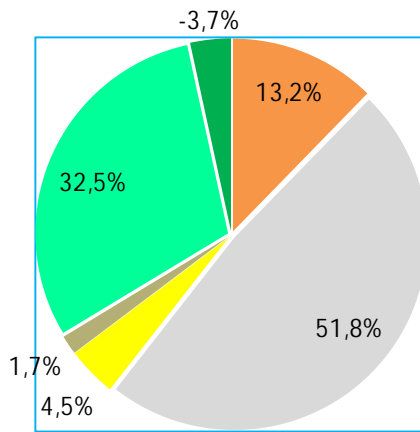
Gesamtstromlieferung EVU Markt Kipfenberg
